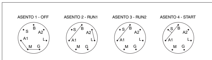
PÄÄKYTKINTEN ASENNOT
