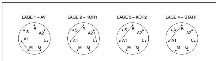
NYCKELBRYTARE, LÅGEN
