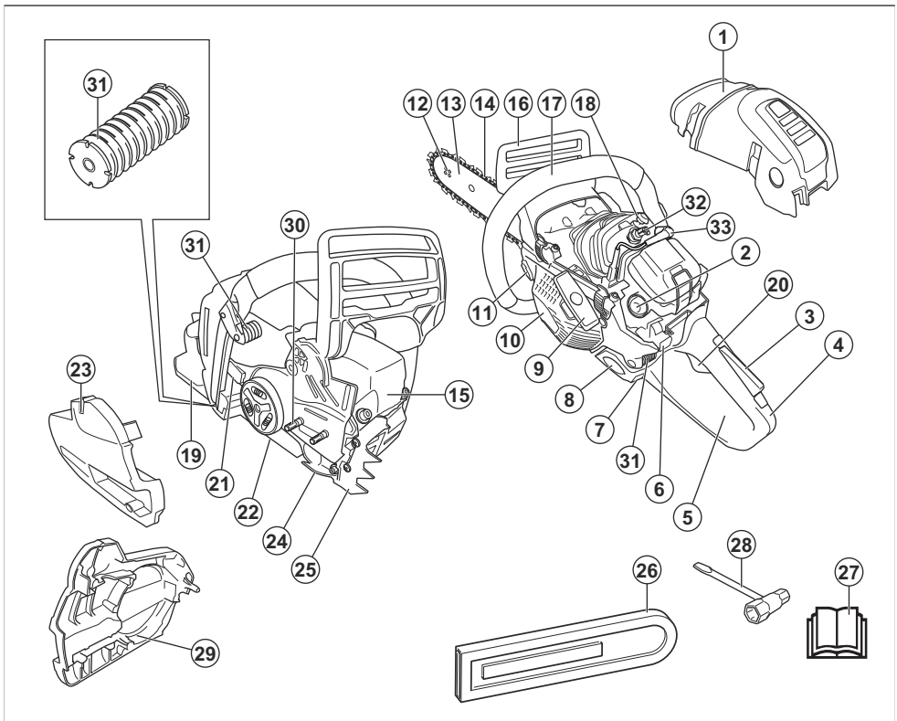
1. Cilinderkap
