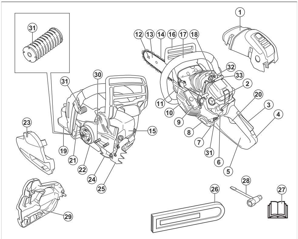
1. Zylinderdeckel
