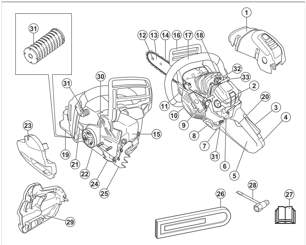
1. Tapa del cilindro
