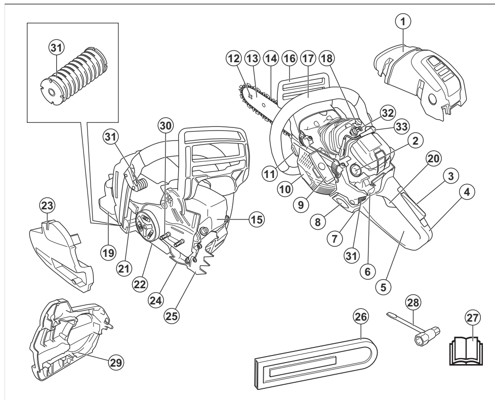
1. Cobertura do cilindro
