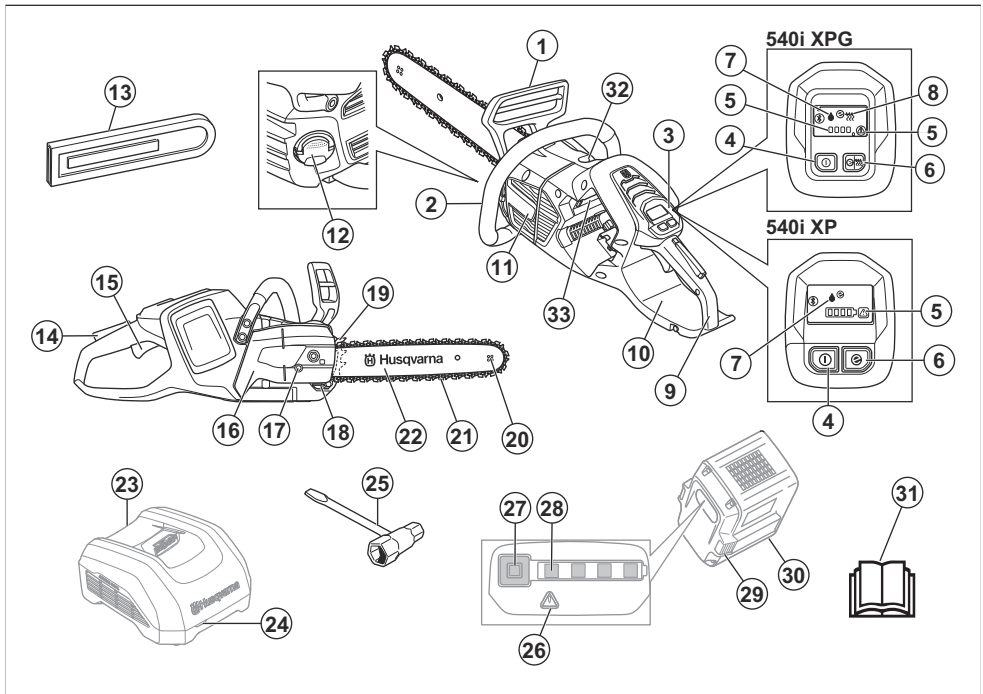
1. フロントハンドガード
