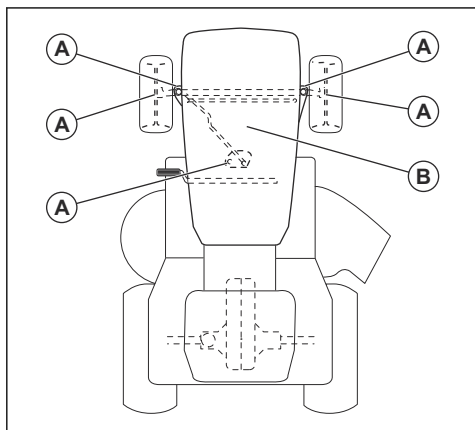
A. Generel smøring. Smør spindlens fedtnippel og tandhjulstænderne på sektorgæaret og ratstammen.
